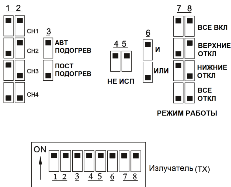
Рисунок 2.11 - Переключатели излучателя
