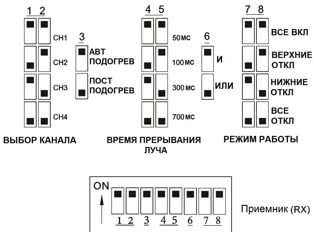
Рисунок 2.12 - Переключатели приемника
